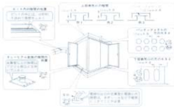
図1-20 キュービクル式高圧受電設備への小動物侵入防止対策例
